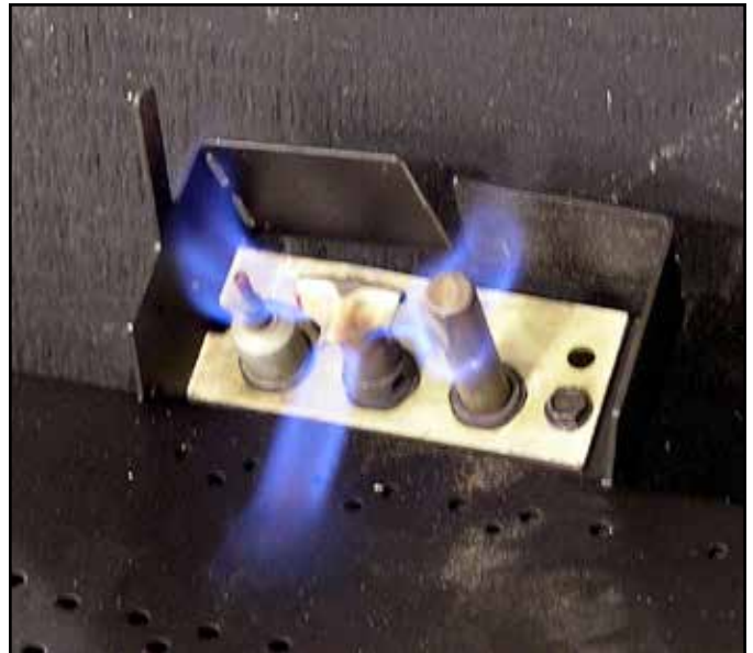
Figure 3.2 Forme de la flamme d'une veilleuse permanente
