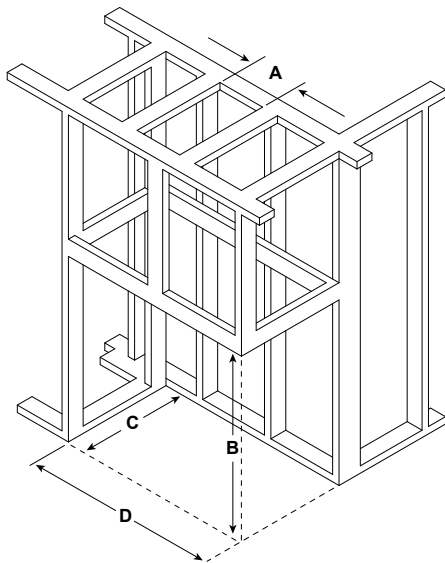
Figure 5.3 Dégagements pour les combustibles
