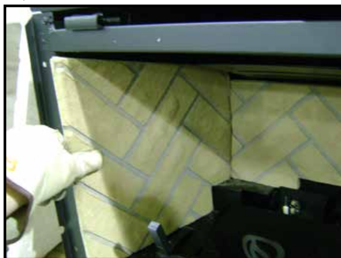
Figure 4. Installation de la brique réfractaire latérale
