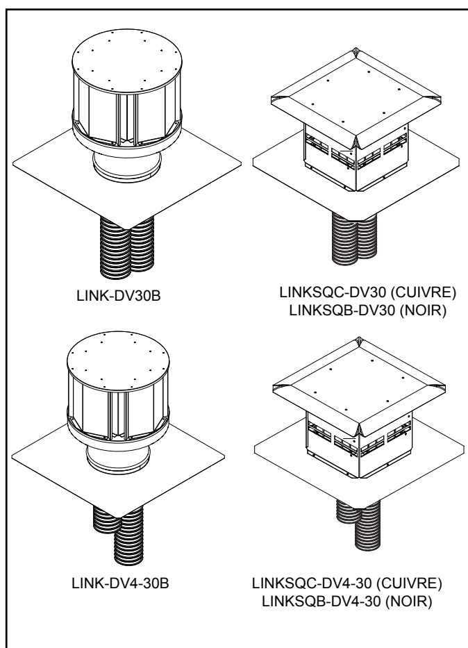
Figure 14.4 Ensembles de doublage de conduit flexible d'évacuation directe
