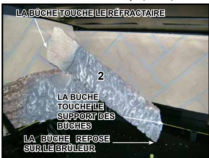
Figure 8. Placer la bûche n° 2
