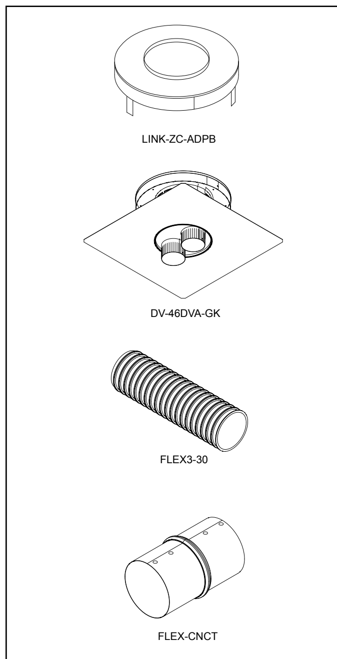
Figure 14.5 Ensembles d'accessoires de doublage de conduit flexible d'évacuation directe
