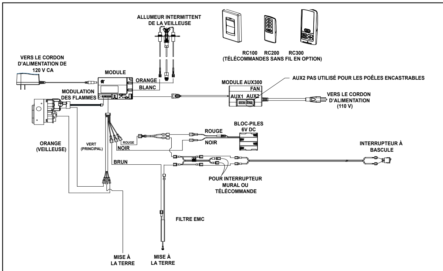
Figure 10.1 Schéma de câblage IPI
