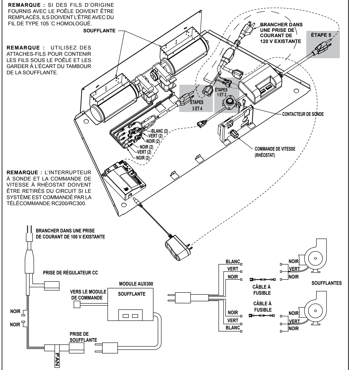
Figure 10.3 Schéma de câblage – soufflante avec télécommande RC200/RC300
