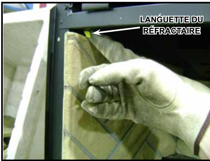
Figure 4. Plier la languette du réfractaire
