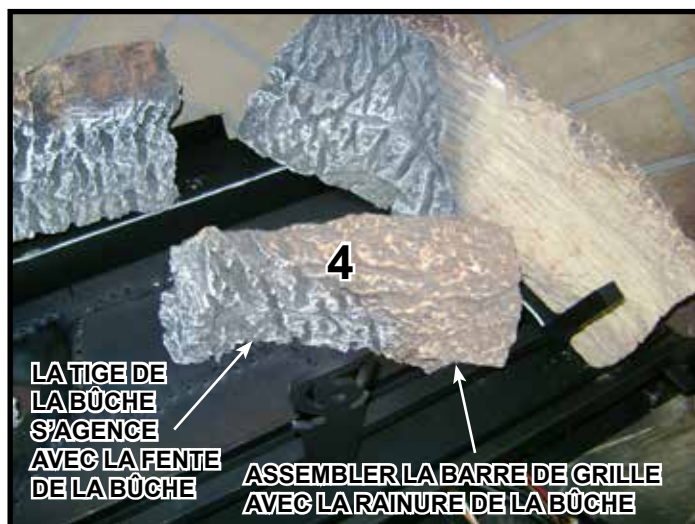
Figure 10. Placer la bûche n° 4
