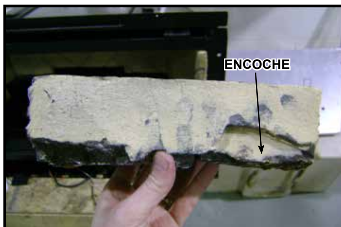
Figure 7. Emplacement de l'encoche sur la bûche n° 1
