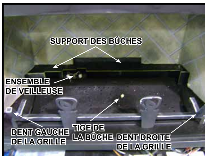
Figure 1. Points de référence pour placer la bûche
