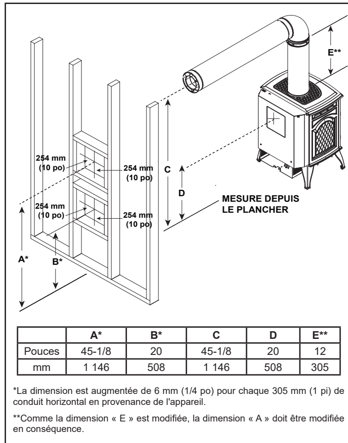
Figure 5.2 Pénétration d'un mur
