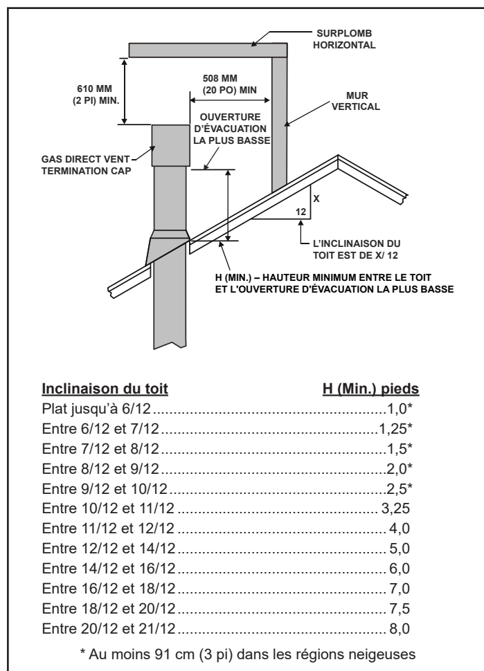
Figure 4.1 Hauteur minimum entre le toit et l'ouverture d'évacuation la plus basse
