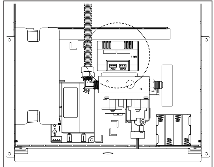
Figure 8.3 Boîte auxiliaire
