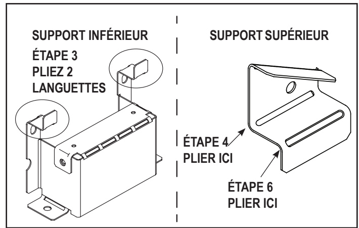
Figure 10.5 Plier le support du réfractaire
