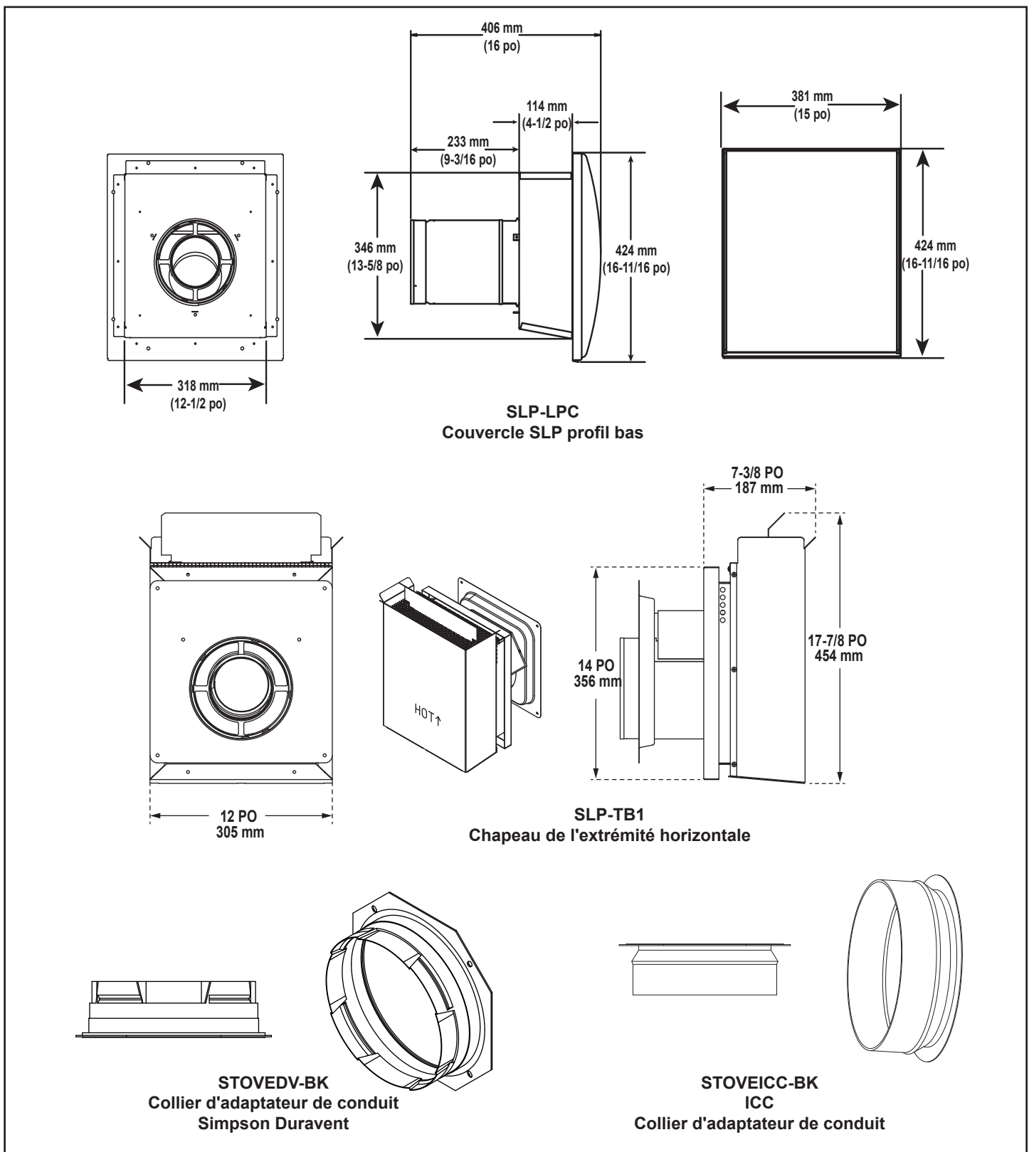
Figure 11.4 Composants du conduit de série SLP
