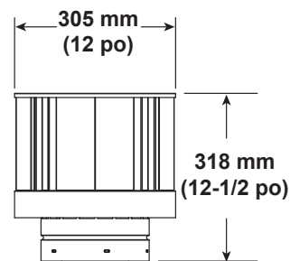
Extrémité de terminal horizontal SLP-TVHW
