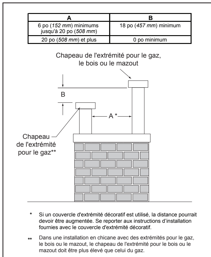
Figure 4.2 Chapeaux de couronne décalés
