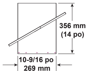
Boîte-support pour plafond cathédrale SLP-CCS-BK – noire
