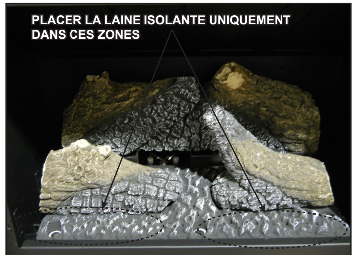
Figure 5. Disposition de la laine isolante
