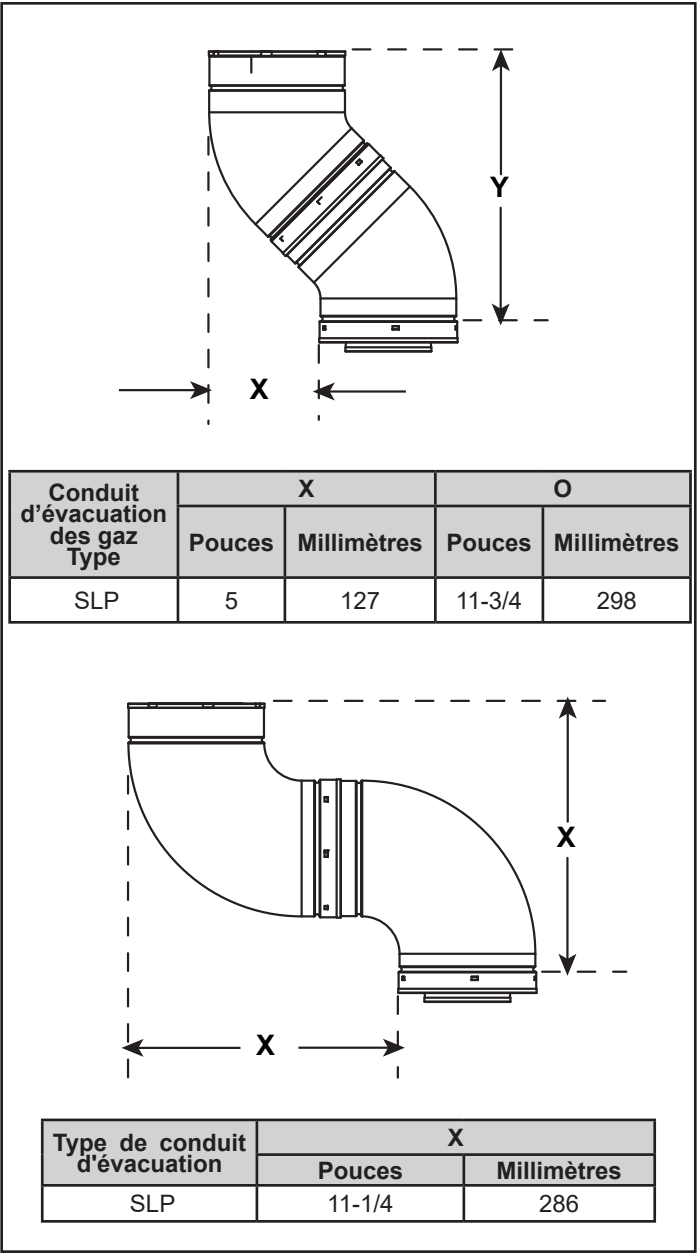
Figure 4.5 Dévoiements verticaux et horizontaux pour les coudes SLP
