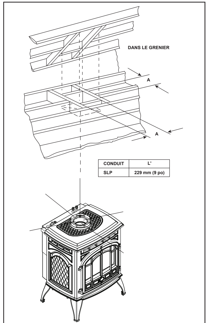
Figure 5.3 Installation du coupe-feu de grenier
