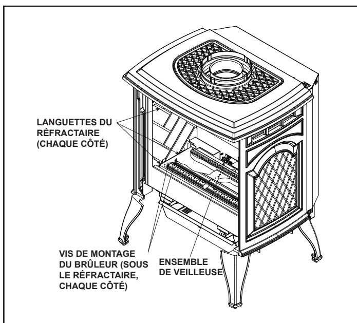
Figure 6.13 Retirer le brûleur
