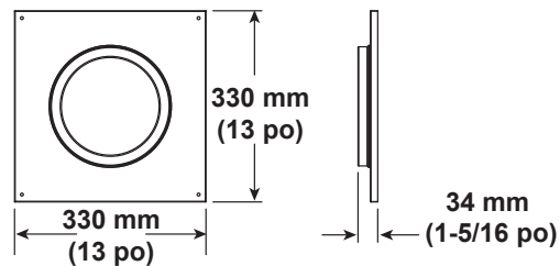
Coupe-feu pour plafond – noir SLP-DCF-BK
