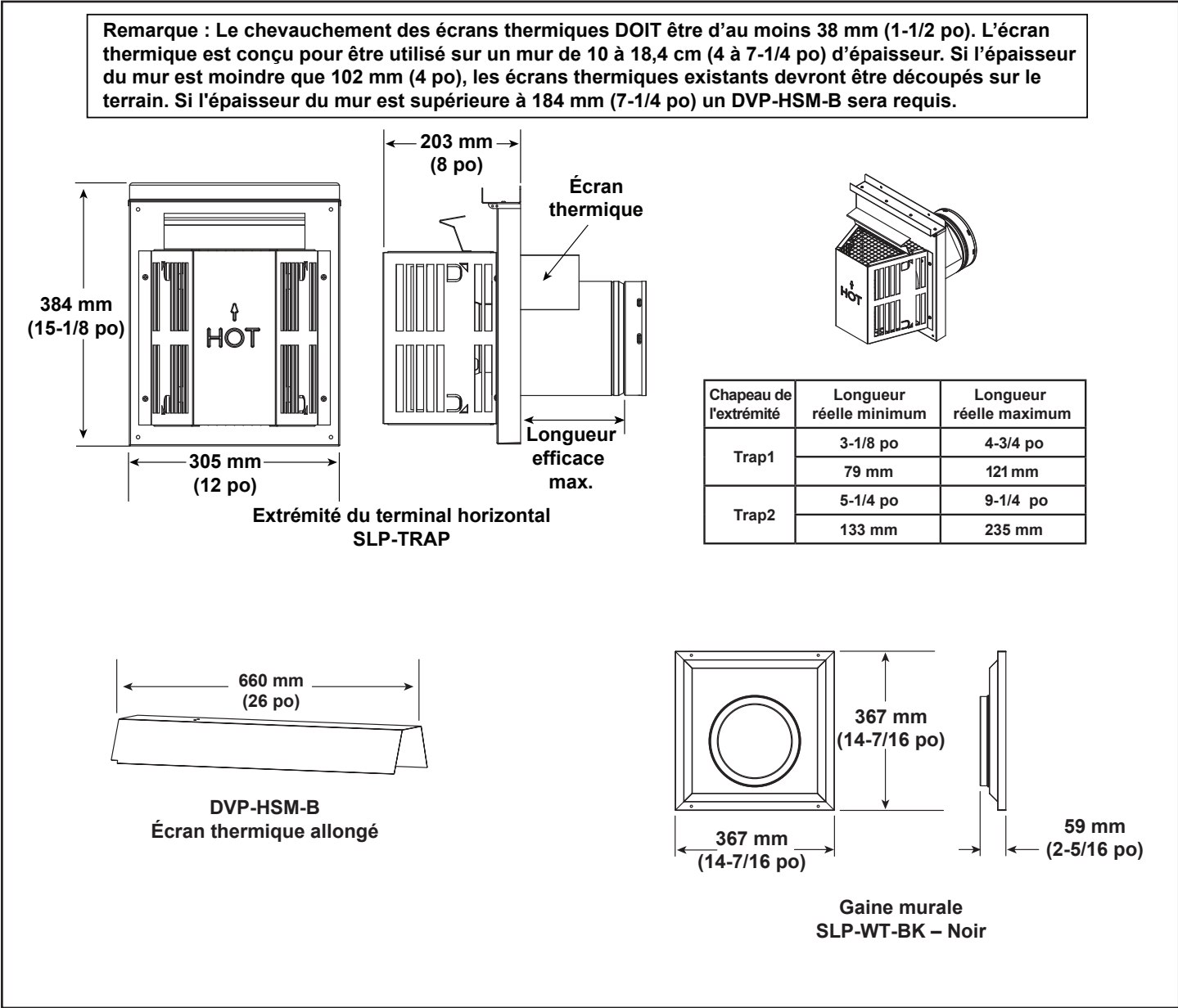
Figure 11.2 Composants du conduit de série SLP
