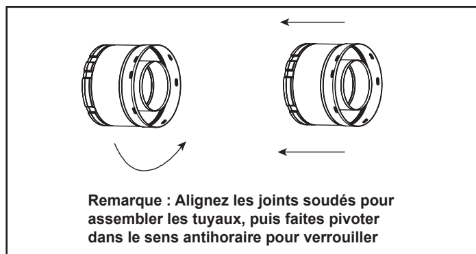
Figure 7.2 Ajout de composants de conduit d'évacuation
