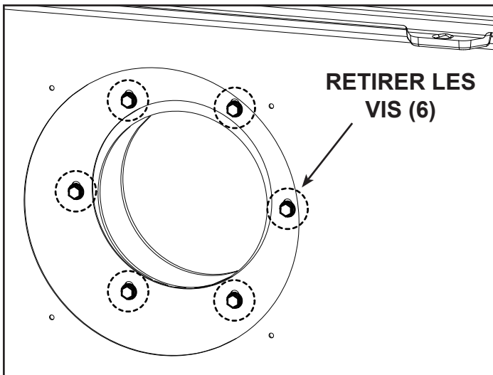
Figure 6.7. Retirer les vis sous la plaque d'accès arrière
