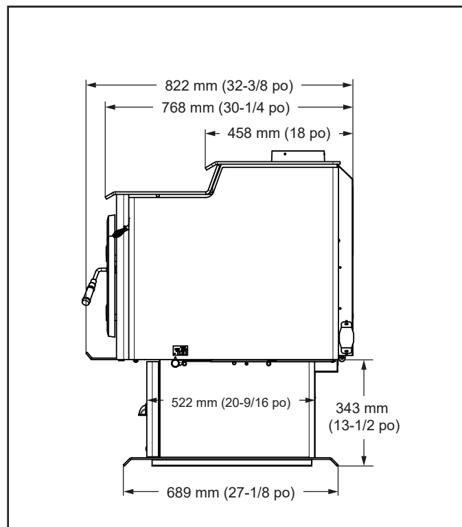
Figure 7.2 Vue latérale
