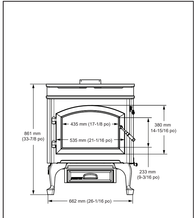
Figure 7.3 – Vue avant
