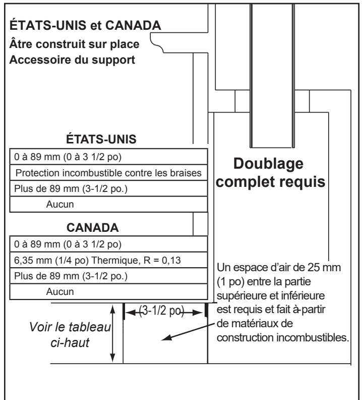
Figure 10.4 - Sans accessoire de support d'âtre réglable
