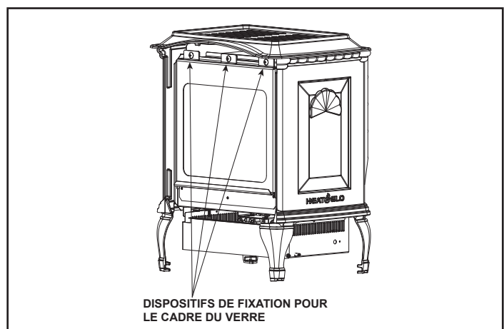
Figure 4.2 Retirer le cadre de la vitre
