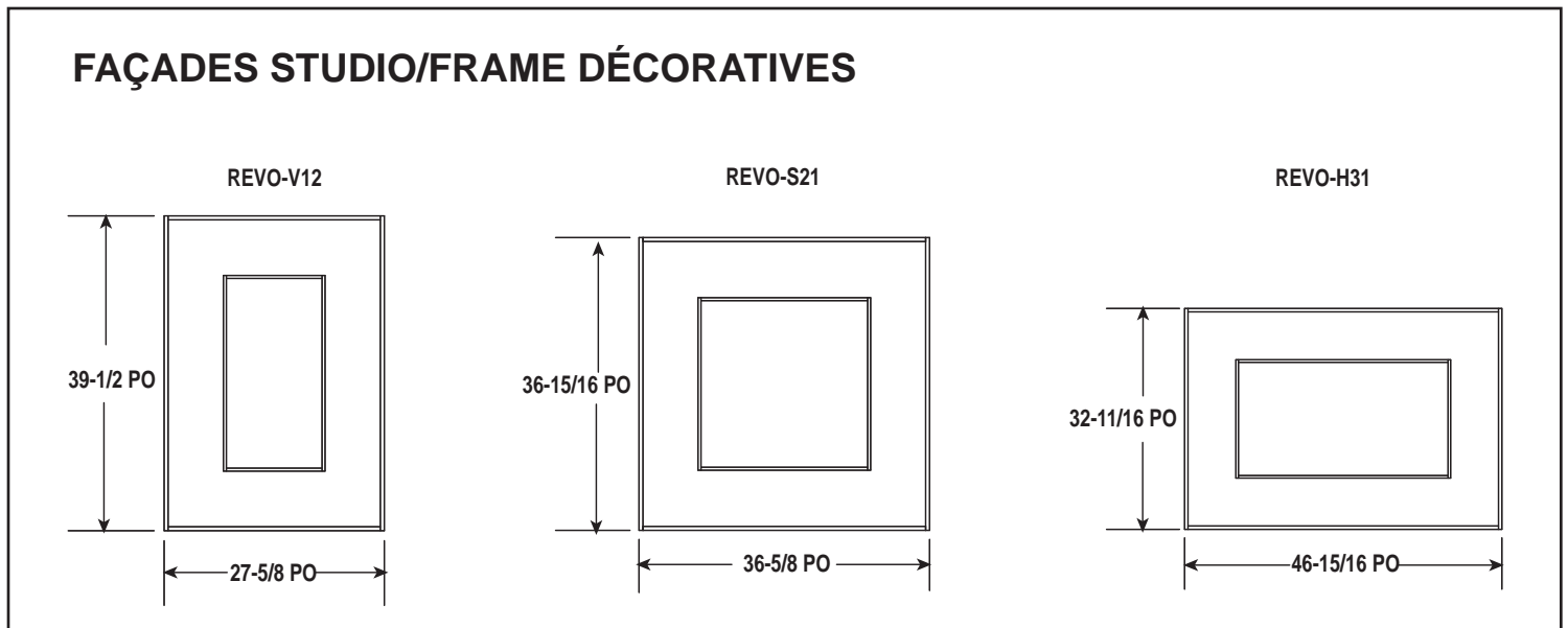
Figure 3.4 Dimensions de l'appareil – Façades Studio/Frame décoratives
