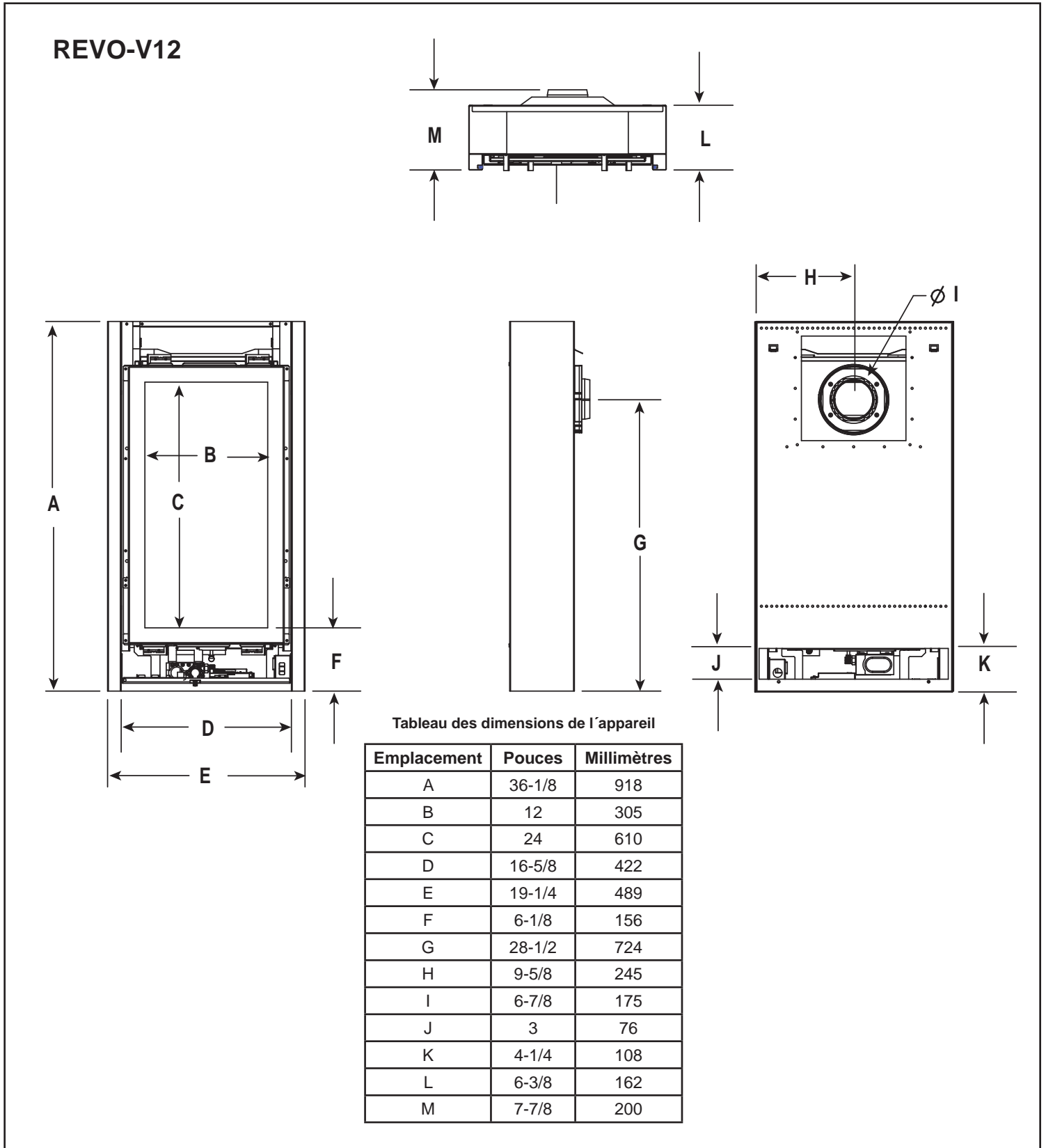
Figure 3.1 Dimensions de l'appareil – Revo-V12
