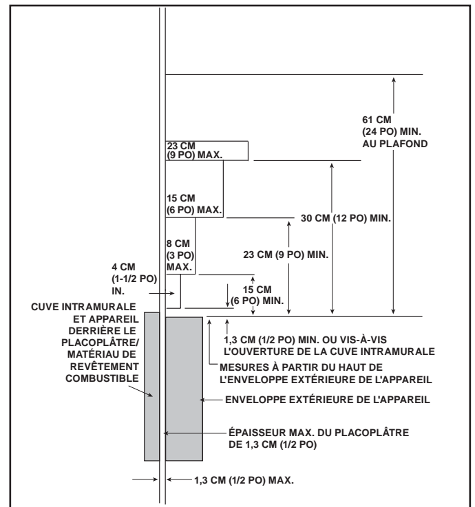
Figure 11.14 Dimensions des combustibles minimaux verticaux et maximaux horizontaux
