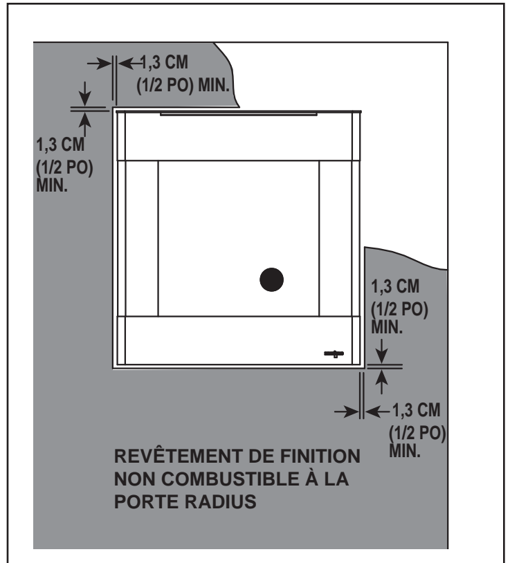
Figure 10.9 Porte Radius – Dégagement par rapport aux matériaux de finition non combustibles
