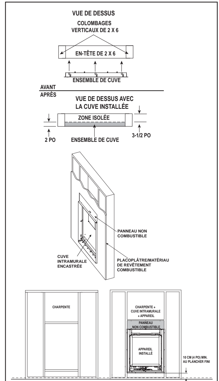
Figure 2.2 Méthode d'installation intramurale
