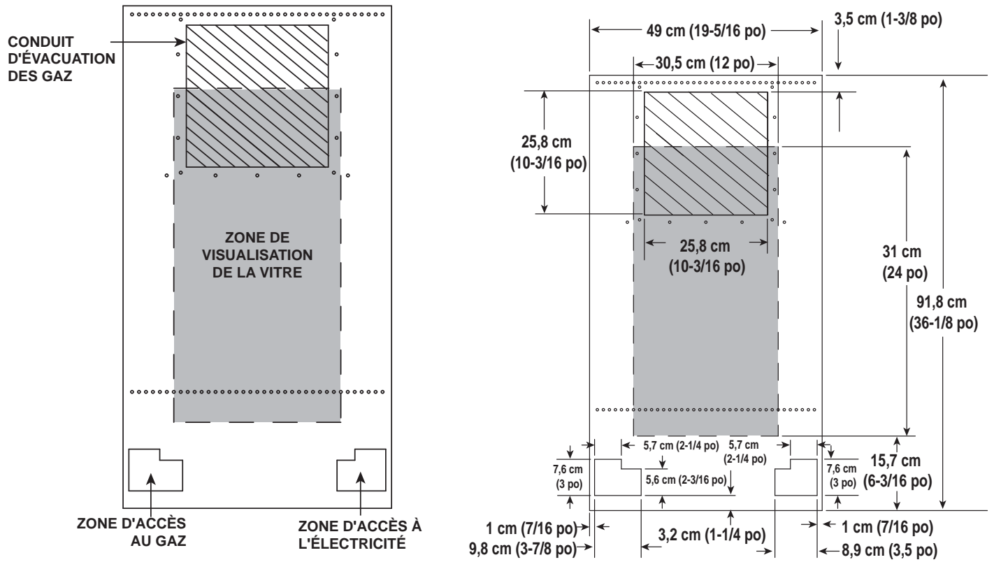
Figure 6.5 Modèle intercalaire de carton de disposition – REVO-V12
