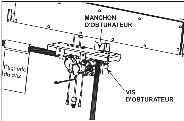
Figure 9.1 Obturateur d'air
