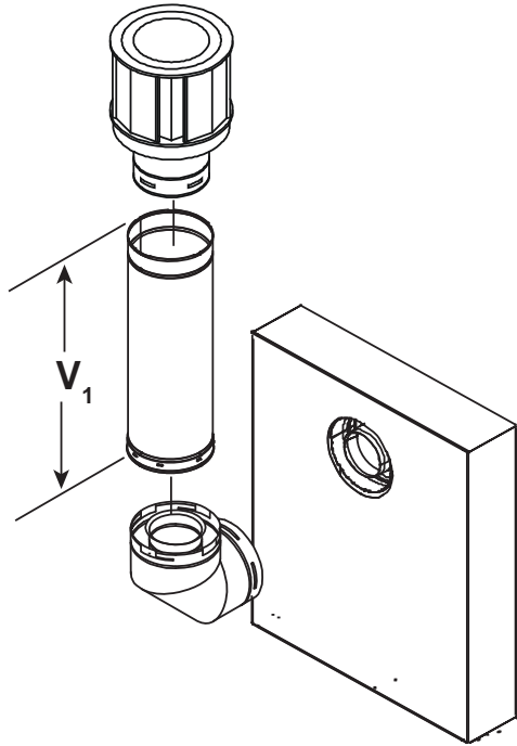
Figure 4.13 Conduit d'évacuation vertical avec un coude
