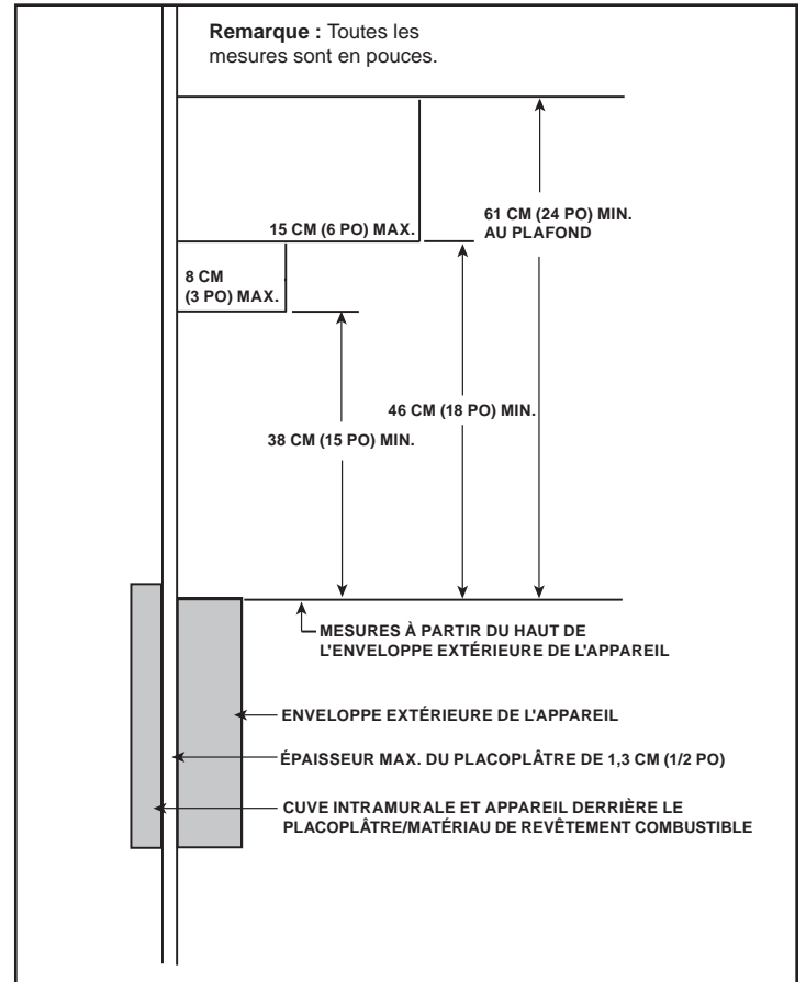
Figure 11.13 Dimensions des combustibles minimaux verticaux et maximaux horizontaux
