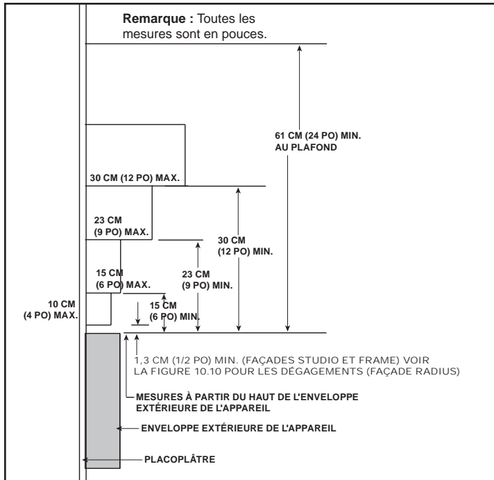
Figure 10.12 Dimensions des combustibles minimaux verticaux et maximaux horizontaux
