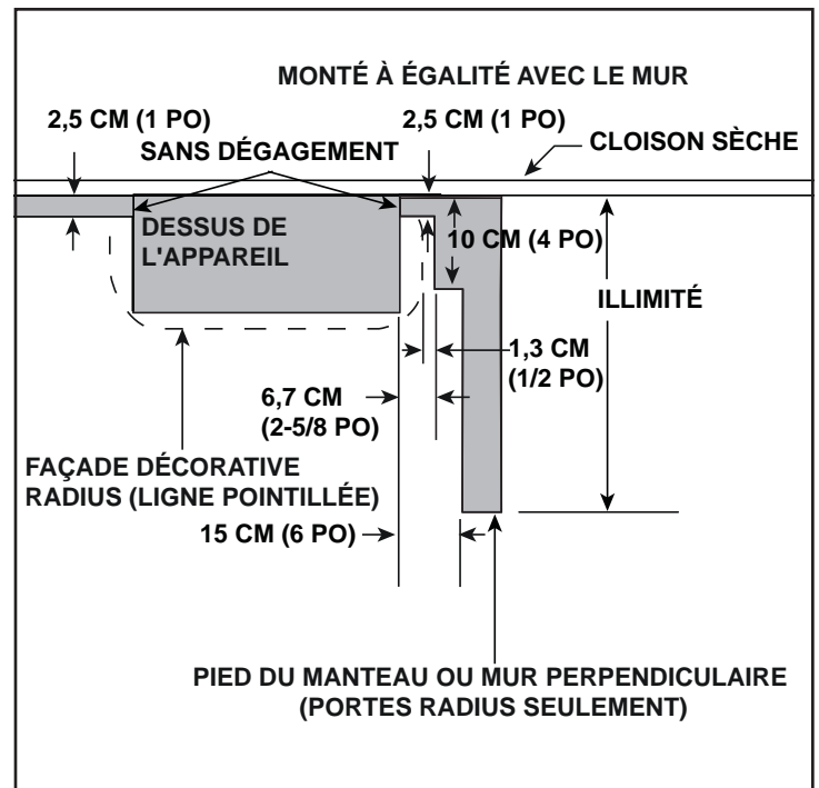
Figure 10.16 Pied du manteau du foyer ou saillie du mur non combustibles (acceptable de part et d'autre de l'enveloppe extérieure)
