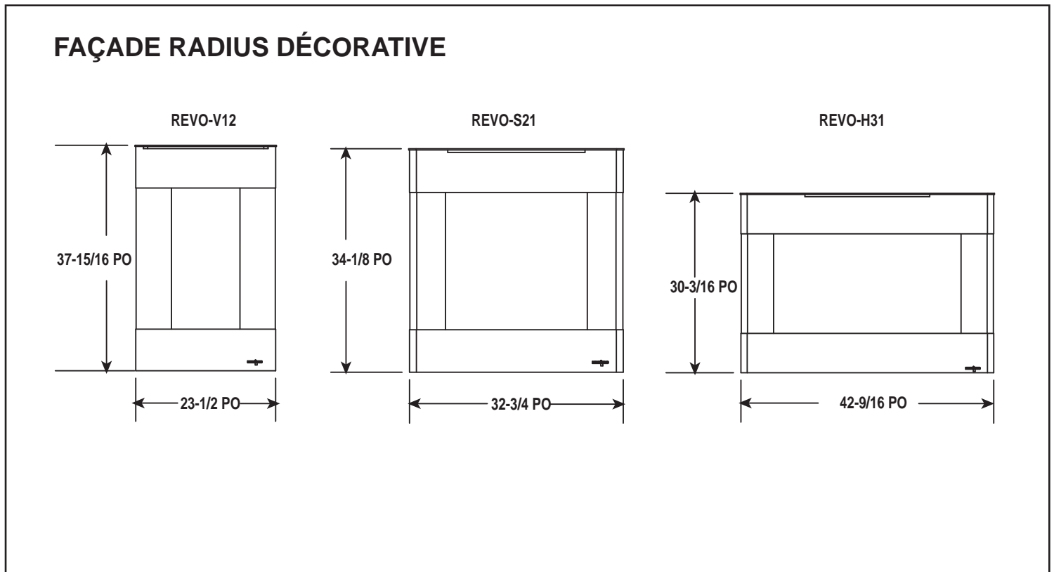
Figure 3.5 Dimensions de l'appareil – Façade Radius décorative
