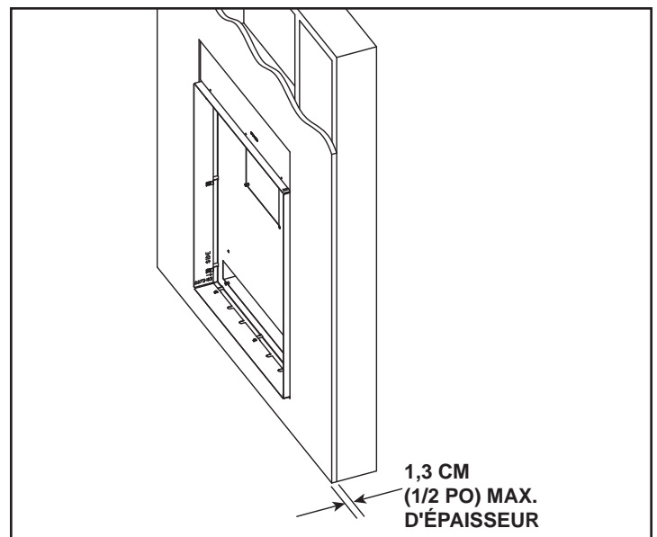
Figure 11.8. Installation de la cuve intramurale – Épaisseur du placoplâtre
