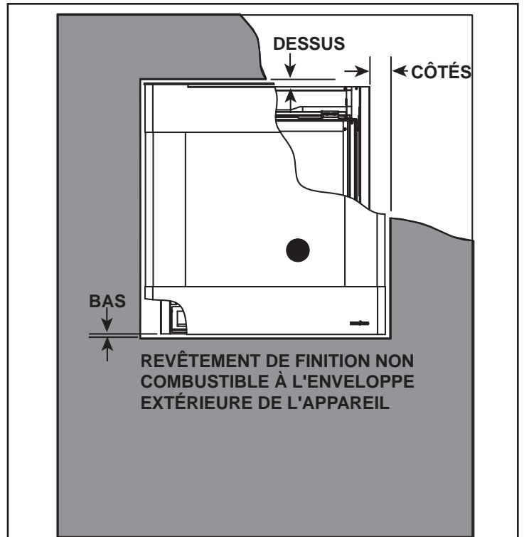
Figure 10.9 Porte Radius – Dégagement par rapport aux matériaux de finition non combustibles
