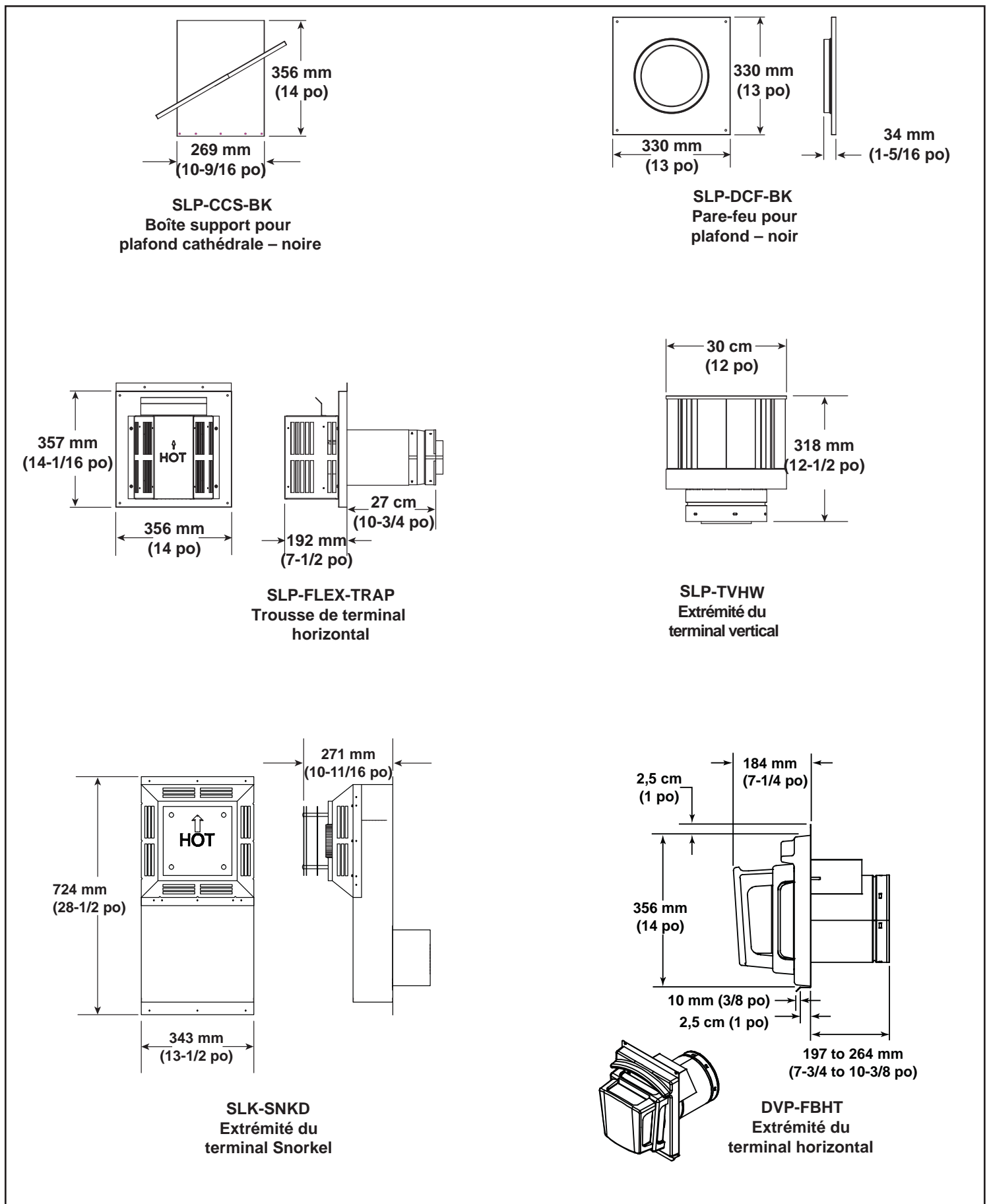
Figure 13.3 Composants du conduit SLP
