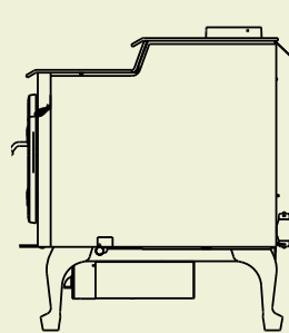
5700 « STEP TOP » » PIEDS STYLE QUEEN ANNE
