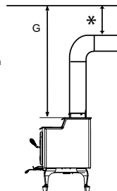
SÉRIE « STEP TOP » Dégagement du foyer au plafond
