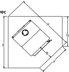
Dimensions pour installation en coin avec tuyau mur simple
