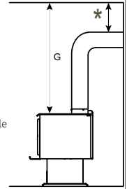
SÉRIE MILLENIUM Dégagement du foyer au plafond
