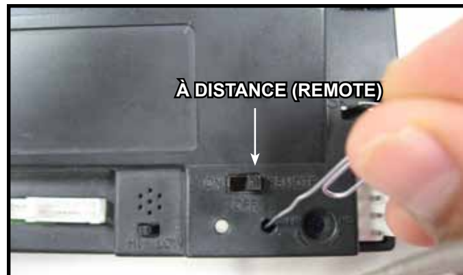
Figure 7. Programmation de la RC300
