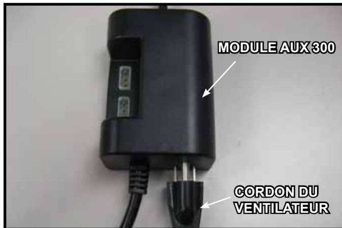
Figure 6. Branchement du ventilateur dans le module AUX300
