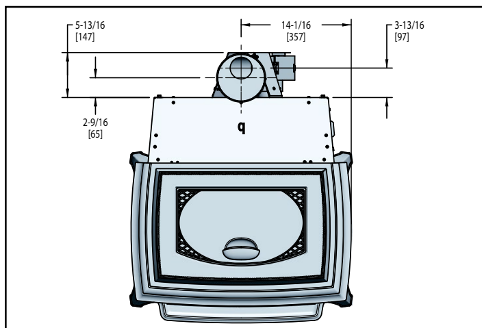
Figure 7.1 – Vue de dessus avec adaptateur supérieur de ventilation et adaptateur de 76 à 152 mm (3 à 6 po)
