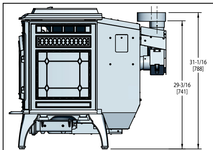
Figure 7.2 – Vue latérale avec adaptateur supérieur de ventilation et adaptateur de dévoiement de 76 à 152 mm (3 à 6 po)
