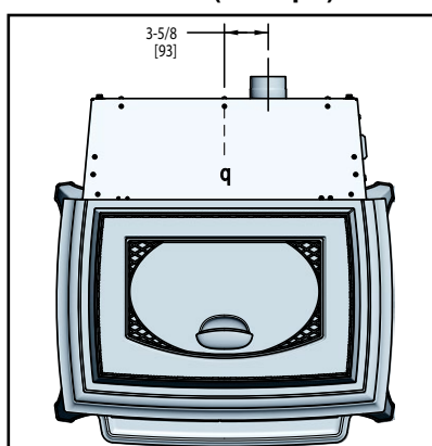
Figure 7.3 – Vue de dessus
