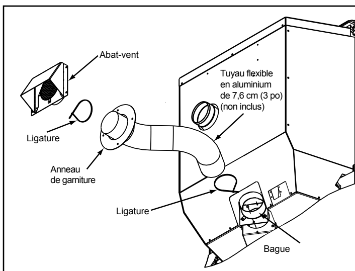
Figure 17.4 - Vue éclatée OAK
