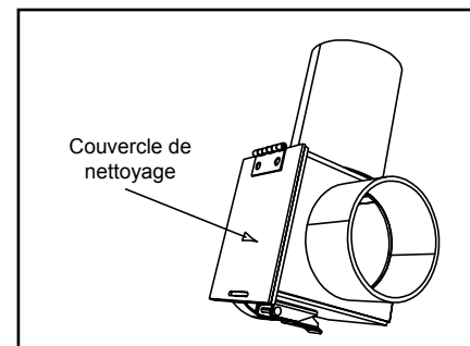
Figure 18.4 – Adaptateur supérieur de ventilation arrière – 90°
